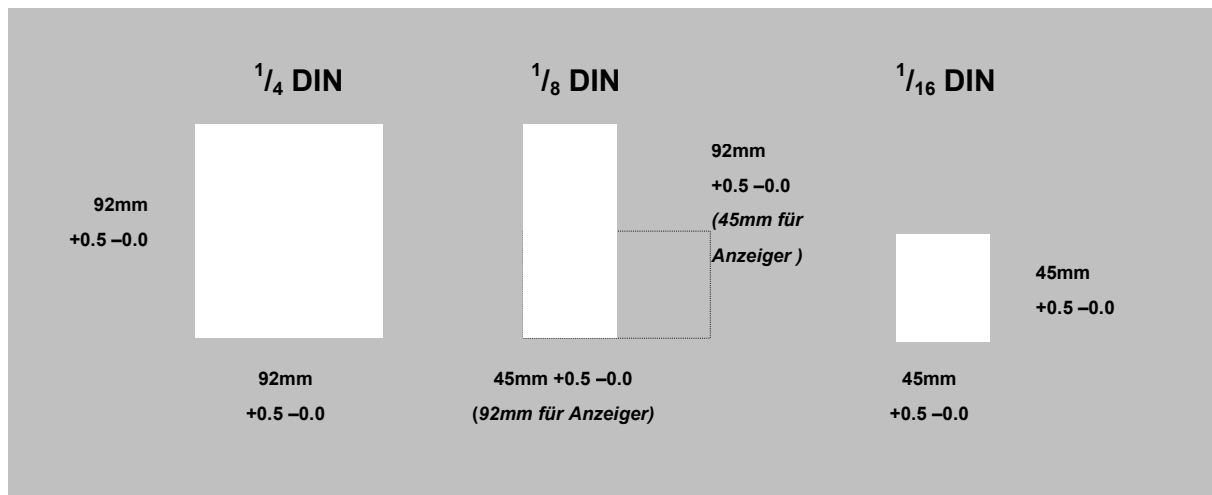
Bild 2 - Montageöffnungen
